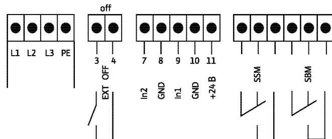
Схема подключения
