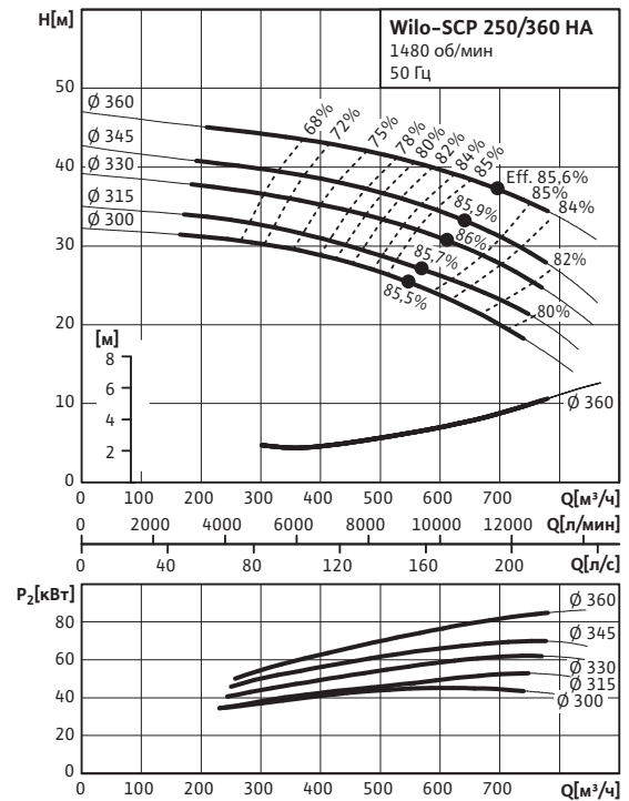
Wilо-SCP 250/360 HA
