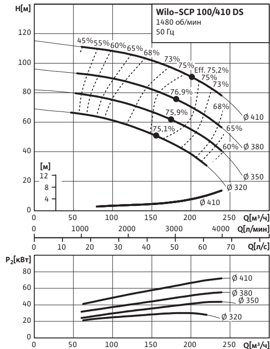
Wilo-SCP 100/410 DS
