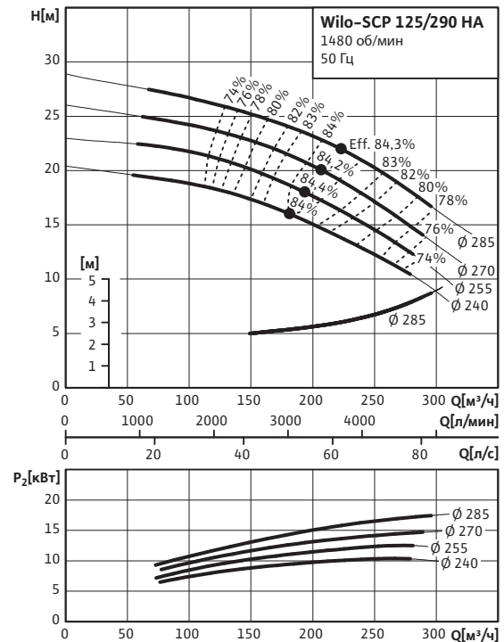
Wilo-SCP 125/290 HA
