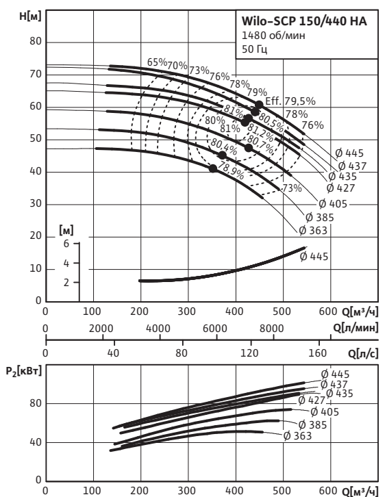
Wilo-SCP 150/440 HA
