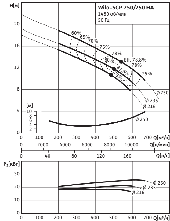
Wilо-SCP 250/250 HA
